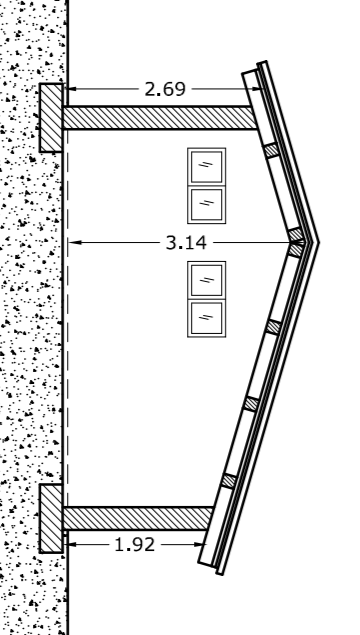
Sezione < X-X' >
