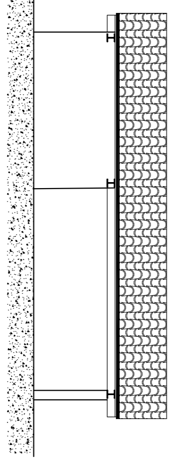
Prospetto < Sud-Ovest >
